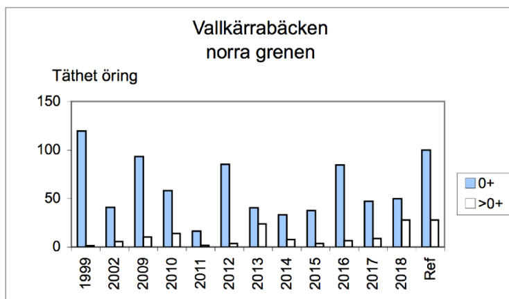
Figur 2. Täthet av öring (antal/100 m 2 ) fångad vid elfiske på lokalen i norra grenen i perioden 1999-2018. 0+ anger årsungar och >0+ äldre öring. Ref. anger elfiskeregistrets jämförvärde (tabell 1).
