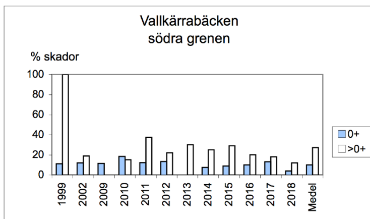
Figur 3. Öring med skador (%) på lokalen i södra grenen i perioden 1999-2018. 0+ anger årsungar och >0+ äldre öring. Medel anger medelvärde för perioden 1999 – 2018.
