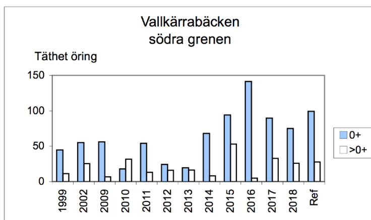
Figur 1. Täthet av öring (antal/100 m 2 ) fångad vid elfiske på lokalen i södra grenen i perioden 1999-2018. 0+ anger årsungar och >0+ äldre öring. Ref. anger elfiskeregistrets jämförvärde (tabell 1).
