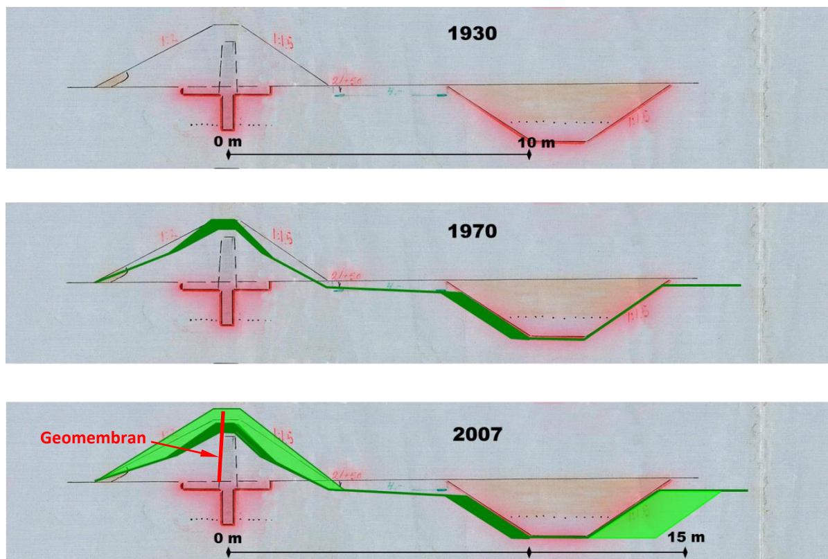
Figur 32. Exempel på en vällanläggning med restaureringsbehov efter ca 40 år.
