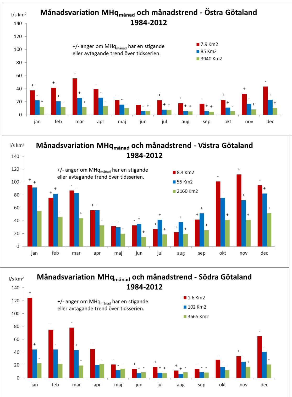
Figur 23. Månadsvariation och månadstrend under perioden 1984-2012 för avrinningsområden med varierande storlek inom östra-, västra- och södra Götaland.
