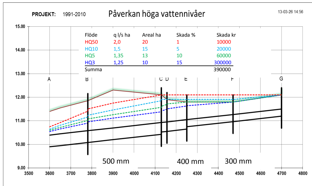
Figur 31 b. Rörledning anlagd år 1960 belastad med 25-35 % högre flöden.
