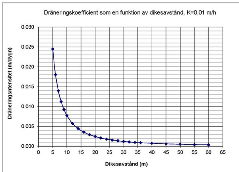
Figur 30. Dräneringsintensiteten som funktion av dikesavståndet för täckdikning av en finmojord eller en aggregerad lera med grundvattenytan 0,4 m under markytan. (Ingrid Wesström, SLU)
