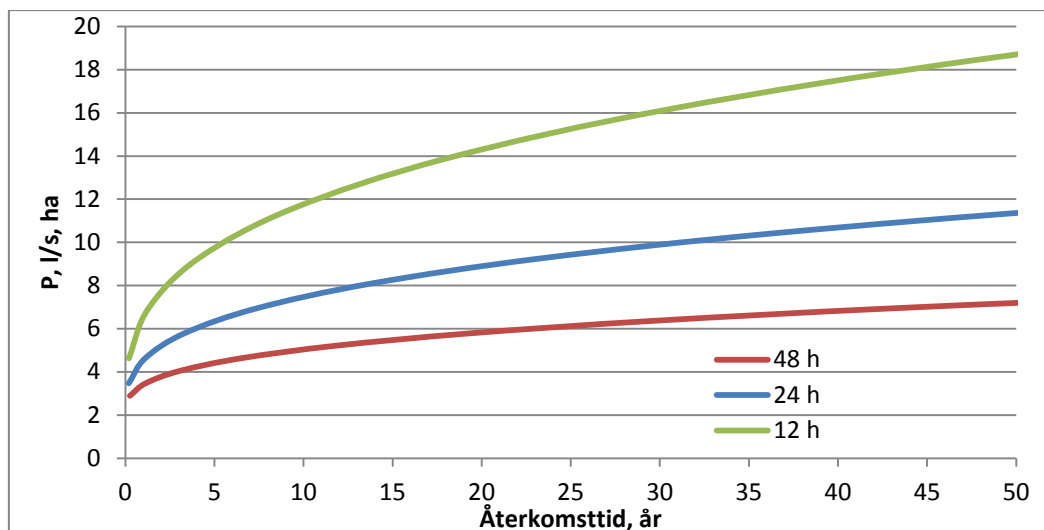
Figur 20. Återkomsttid och regnintensitet för nederbörd med varaktigheten 12, 24 och 48 timmar. Beräknat enligt P 104, (Svenskt vatten, 2011:1)
