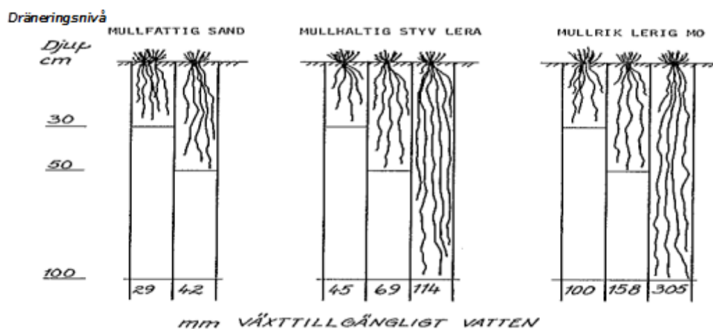
Figur 8. Växttillgängligt vatten och rot djup som funktion av dräneringsnivå och jordart, Johansson och Linnér SLU (1977).
