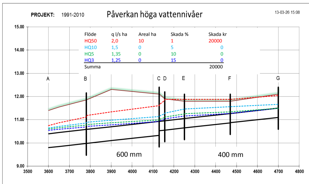
Figur 31 c. Rörledning, uppdimensionerad för 25-35 % högre flöden.
