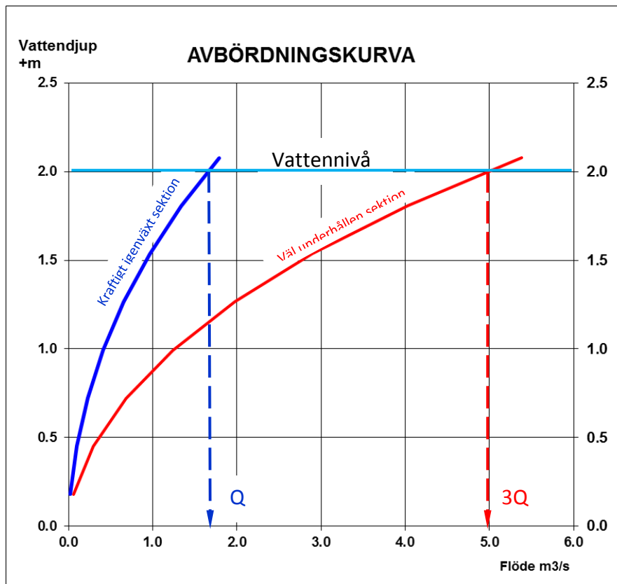
Figur 19. Avbördningskurva utvisande förhållandet mellan vattendjup och flöde dels för en sektion med underhållsbehov, dels för en väl underhållen sektion. Kapaciteten är 3 gånger större i den underhållna sektionen. För dimensioneringen är det vattennivån som är avgörande.
