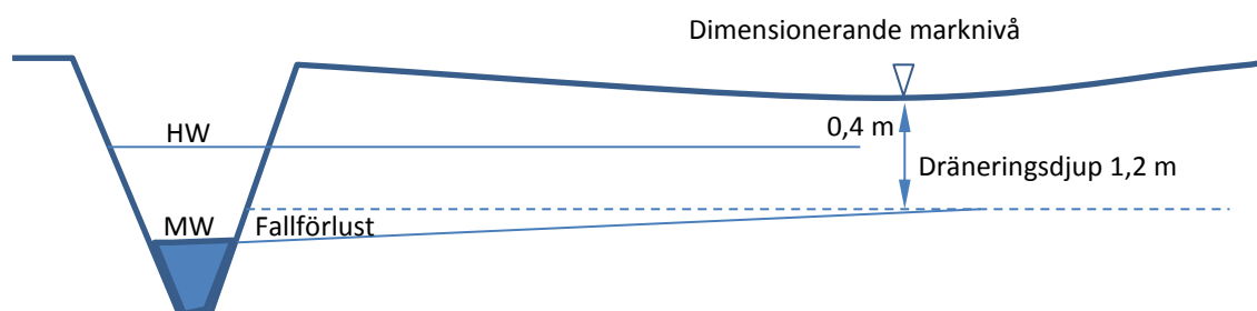
Figur 27. Dimensionerande nivåer för en vattenanläggning.
