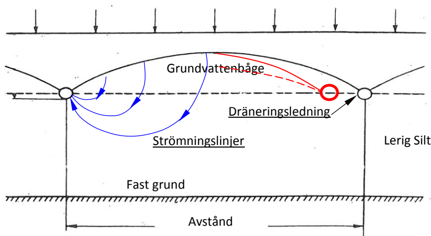
Figur 29. Dränering med täckdiken, strömningslinjer och grundvattenbåge vid minskning av dikesavståndet (Vattenenheten).
