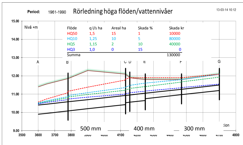
Figur 31 a. Rörledning anlagd år 1960 enligt nuvarande dimensioneringsnivå.
