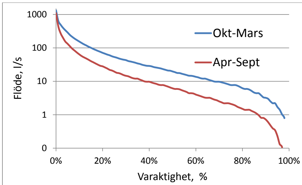
Figur 15. Varaktighetsdiagram för sommar- resp. vinterperioden för ett vattendrag i Östergötland. Observera att skalan är logaritmisk.
