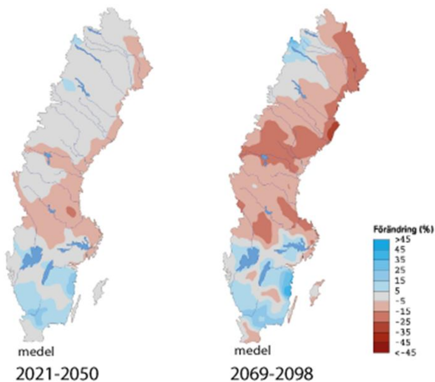
Figur 25. Förväntad utveckling av flödeshändelser med 100-års återkomsttid (SMHI)
