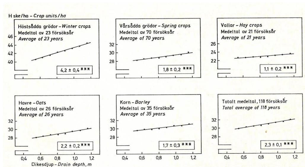
Figur 9. Avkastningsökning relativt dräneringsdjup för olika grödor (Håkansson, 1969)
